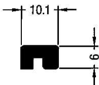
Fixierprofil
