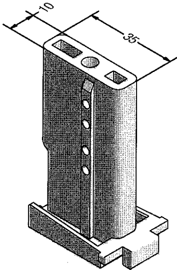
Mechanischer Verbinder Sposse 68
