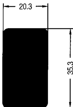
Mechanischer Verbinder universal für Pfosten 78
