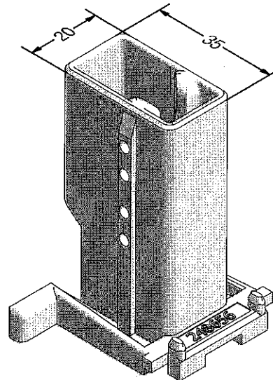
Mechanischer Verbinder Pfofen 78 BT60
