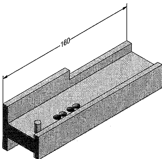
X Bohrlehre Pfosten/Sprosse
