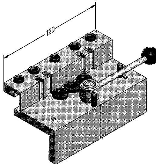
Bohrlehre Blendrahmen für Pfosten 78
