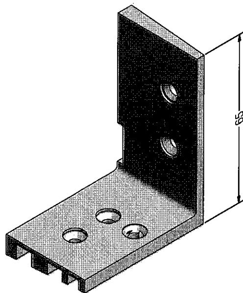
Sprossenwinkel für Sprosse 68 TD
