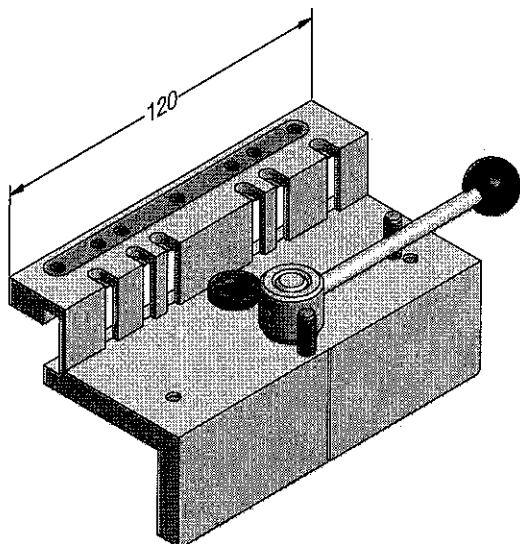
Bohrlehre Blendrahmen für Sprosse 68
