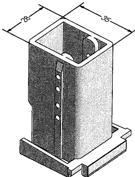
Mechanischer Verbinder Pfofen 86
