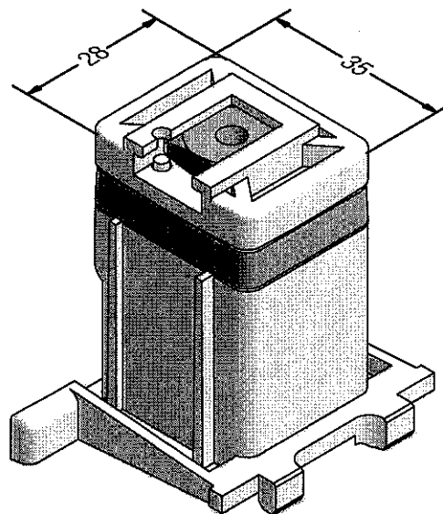
Mechanischer Verbinder mit Dichtkissen Pfofen 86
